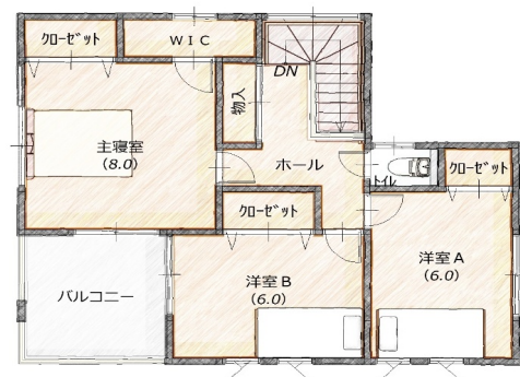
2F プラン
